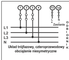
miernik 3V 96x96mm
